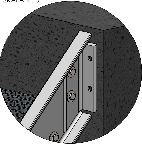
SZCZEGÓŁ B SKALA 1 : 5
